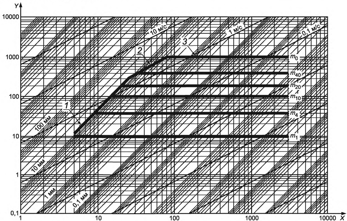
Рисунок 2 — Типичные характеристики электродинамического вибростенда
