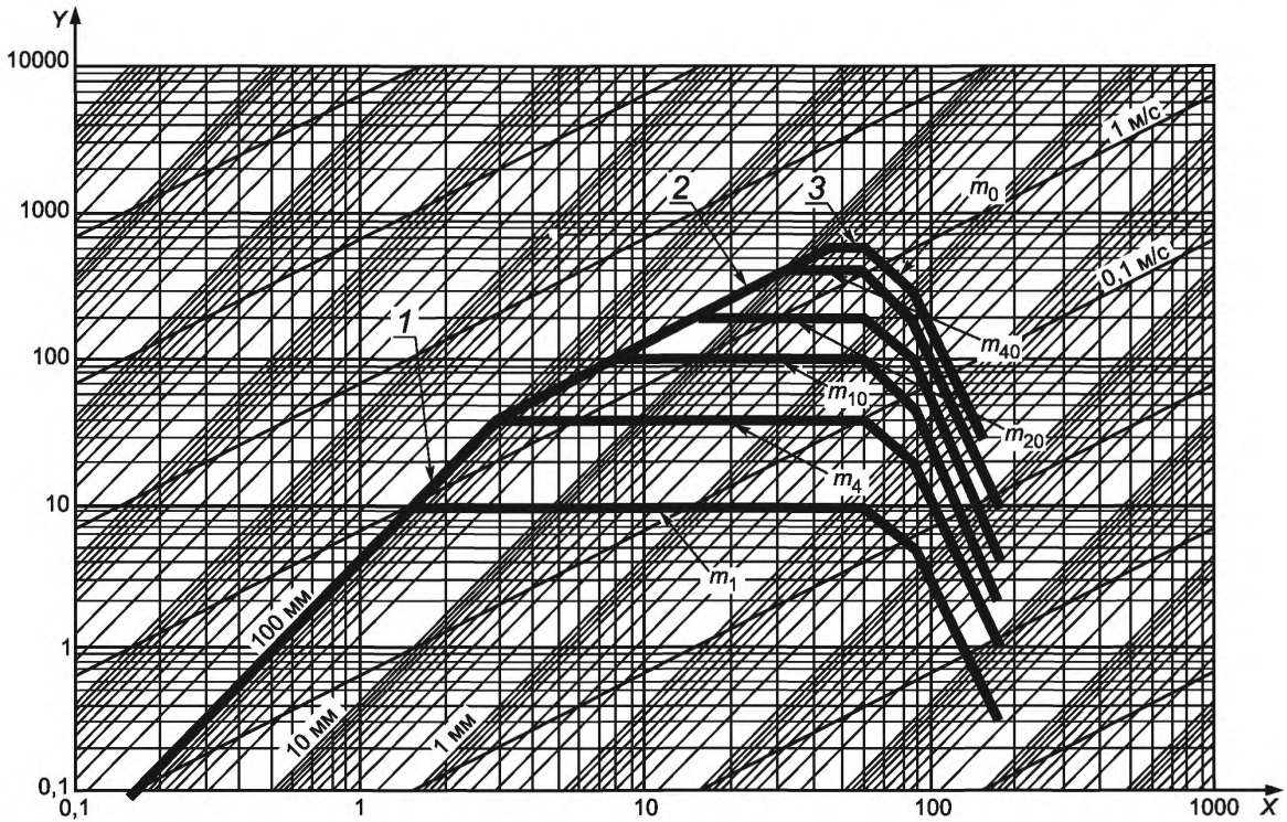
Рисунок 4 — Типичные характеристики гидравлического вибростенда
