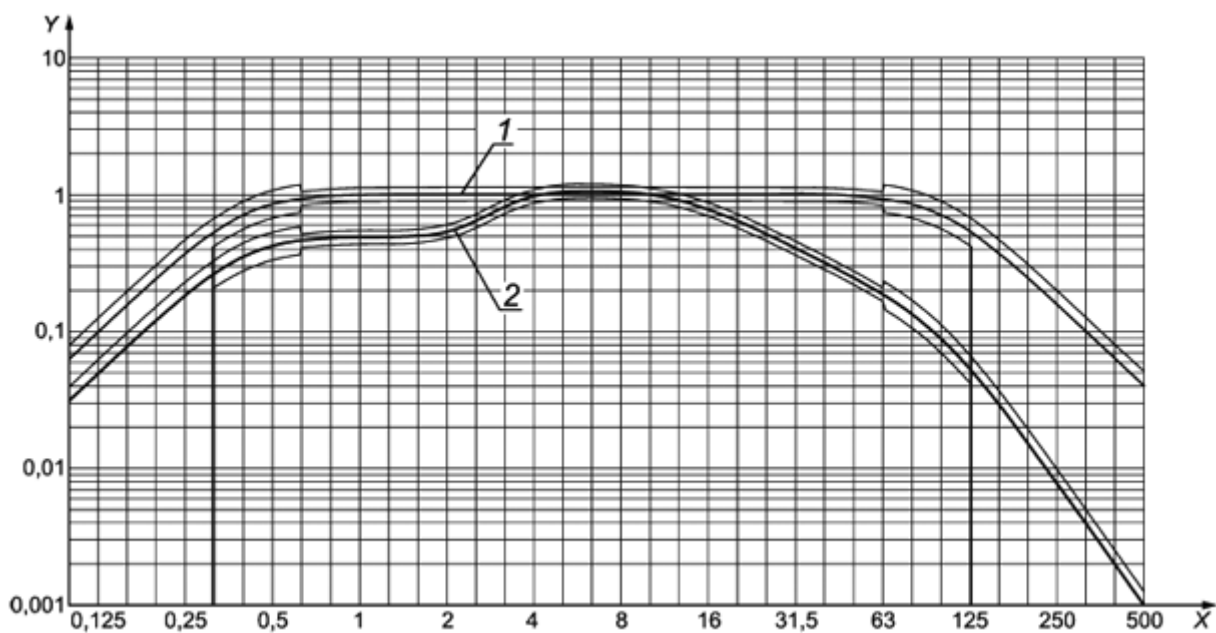
X - частота, Гц; Y - модуль частотной характеристики; 1 - полосовой фильтр; 2 - функция частотной
